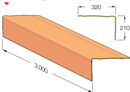
scossalina angolare in polimglass
